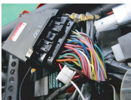
配線の接続先は、シート下のECU、白2Pカブラーとバッテリーマイナス端子。
