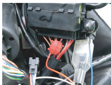
配線の接続先は、ECUカプラーおよびヒューズボックスの配線。
