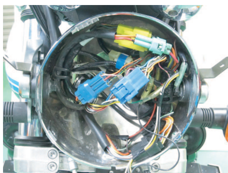
配線の接続先は、ヘッドライトケース内の配線およびサイドカバー内のカブラー。
