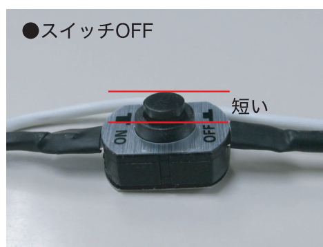
②ON/OFFスイッチ（部品表⑩）の白線のオスギボシを接続します。
