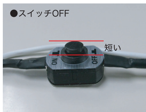
②ON/OFFスイッチ（部品表⑥）の白線のオスギボシを接続します。
