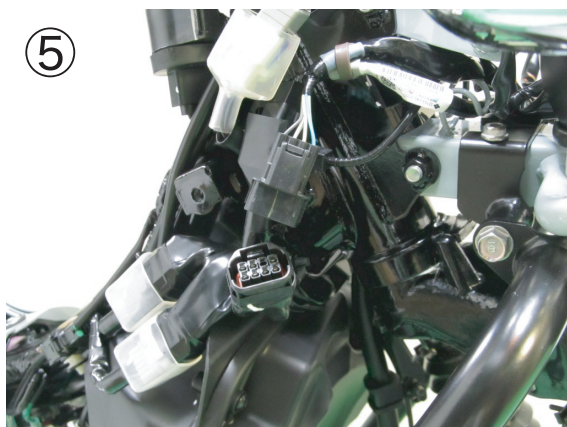
⑤ ノーマルヘッドライトハーネス黒 8 P コネクターを分割します。コネクターは車体右側キーシリンダー下にあります。
