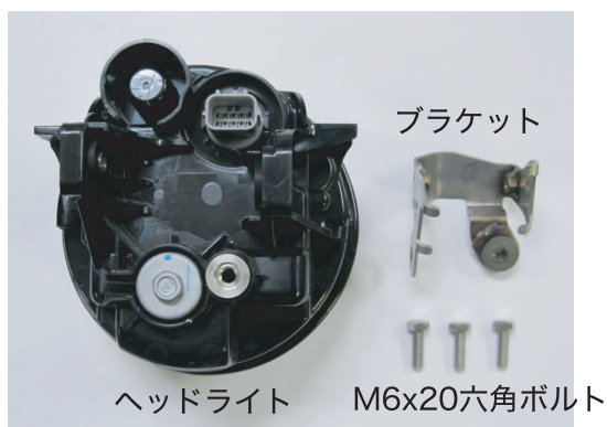
⑤ヘッドライトとブラケットを分割します。 M6x20六角ボルトは2本再使用します。
