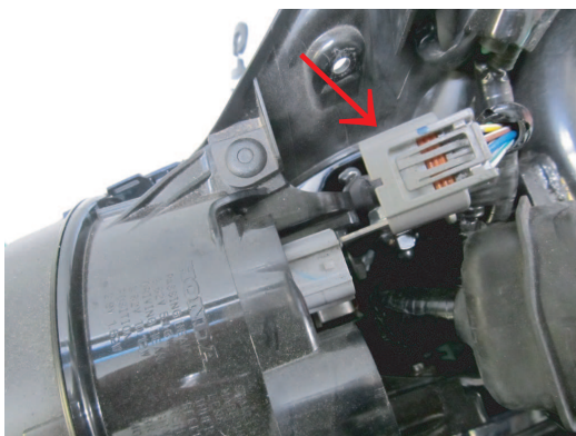
①ヘッドライトユニット後方の灰8P防水カプラーを外します。
