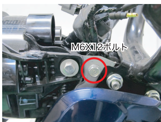
③赤丸のM6X12ボルトを外します。 反対側にも同じボルトがありますので、 合計2本外します。
