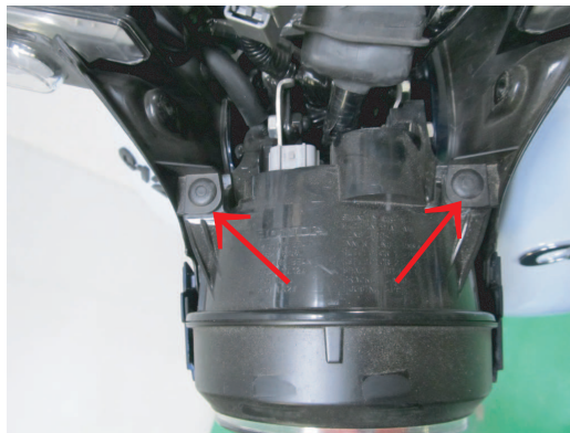
②プッシュリベット2個を外します。 プッシュリベットは再使用しません。
