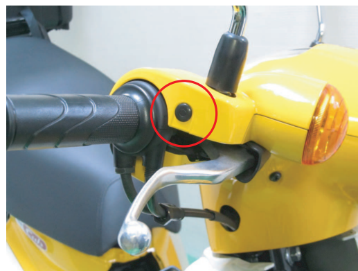
③○で囲った部分のブラリベットを外します・ 中央部分を軽く押して凹めるとロックが外れて ブラリベットを取り外す事ができます。
