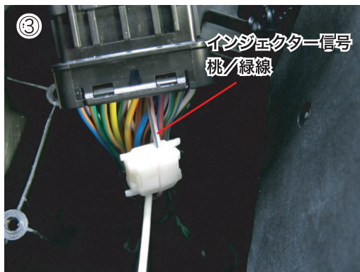
車体側ECUのインジェクター信号……………桃／緑
