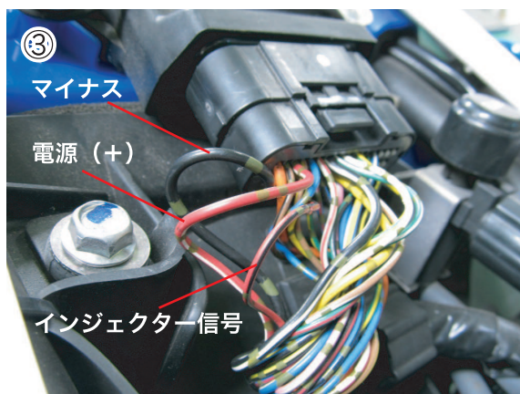
車体側(ECU配線)
